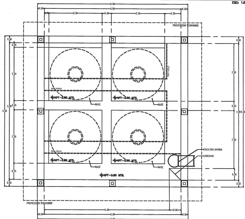
PLANTA GEOMETRICA.
