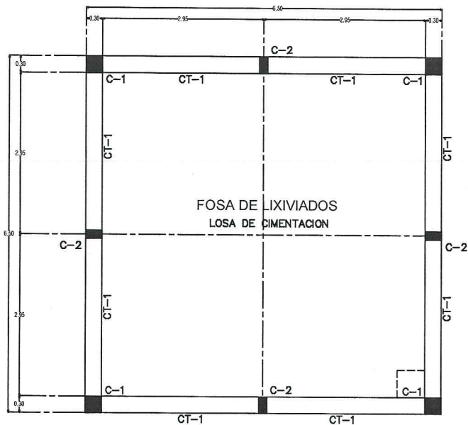
PLANTA DE CIMENTACION.
